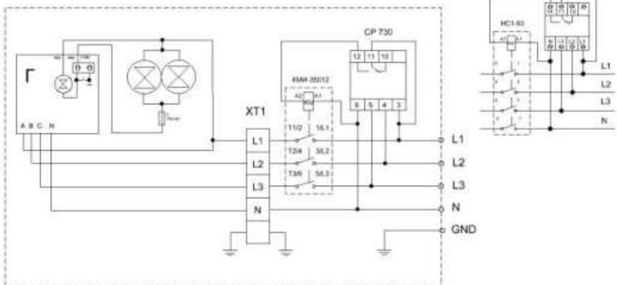
Электрическая схема соединения генератора на 6 кВт ИПВ
