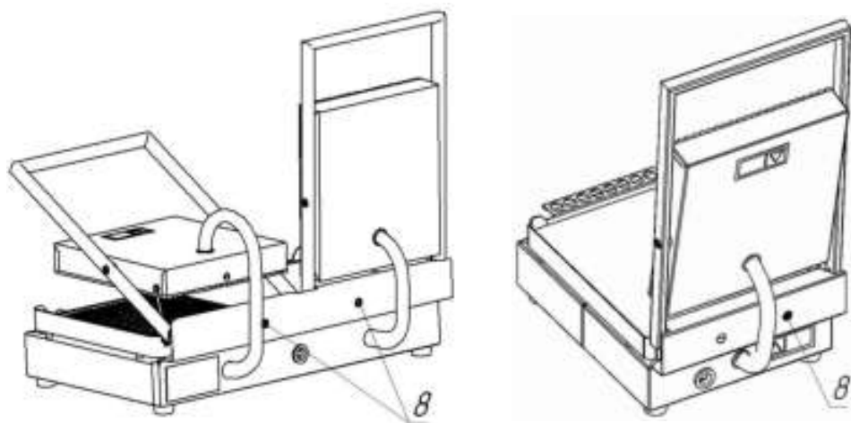
Рис. 2. Общий вид гриля. Вид сзади.
