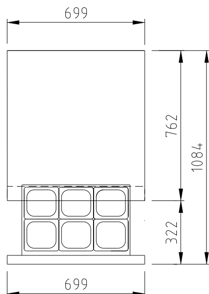
ВИД СВЕРХУ
