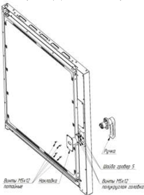
Рис. 5. Замена ручки
