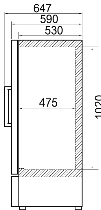
ВИД СБОКУ
