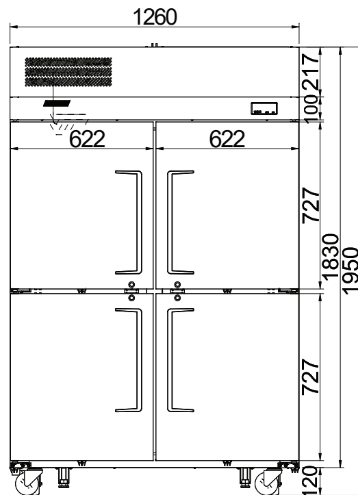
ВИД СПЕРЕДИ
