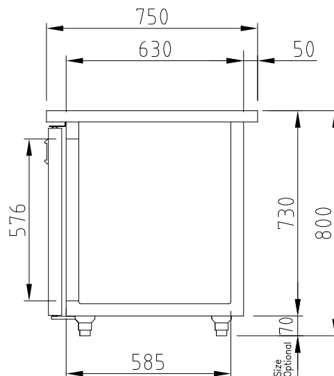
ВИД СБОКУ
