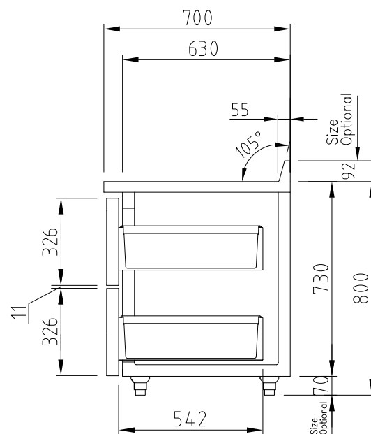
ВИД СБОКУ
