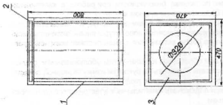
Рисунок 4 - Подставка: 1- уголок 20х30х3; L = 800; 2- уголок 20х30х3; L= 470; 3- уголок 3,5х457х457
