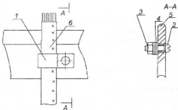
Рисунок 5 - Схема подключения кипятильника к сети; 1 - скоба; 2 - винт; 3 - гайка; 4 - шайба; 5 - кожух; 6 - кабель
