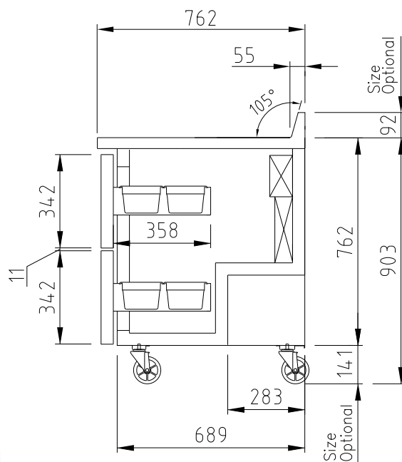
ВИД СБОКУ
