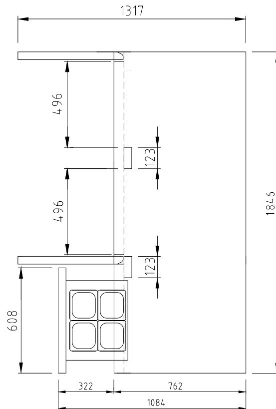
ВИД СВЕРХУ
