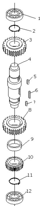
Рис. 3 – Приводной вал
