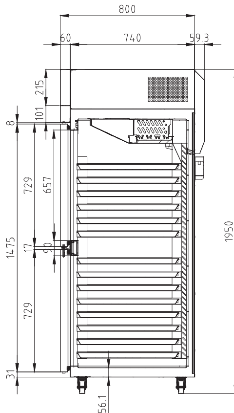
ВИД СБОКУ
