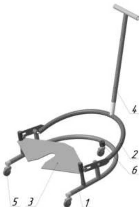
Рисунок 4 – Тележка подкатная
