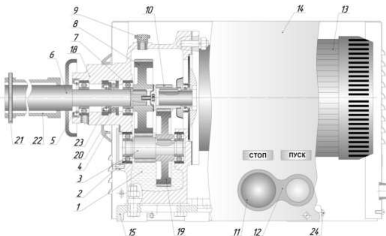
Рисунок 3 – Приводной механизм ПМ
