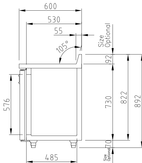
ВИД СБОКУ
