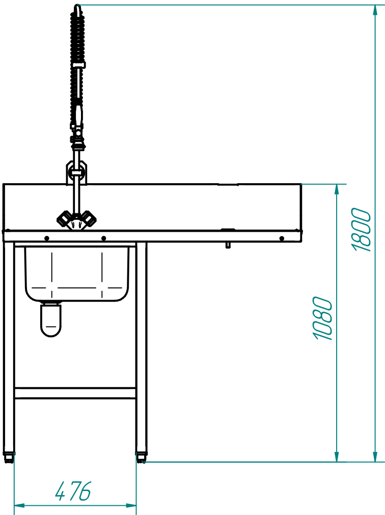
Левое исполнение
