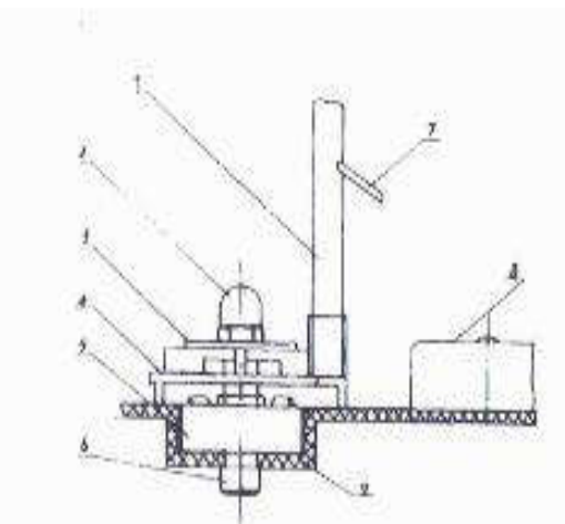
Рисунок 2: Установка узла роздачи
