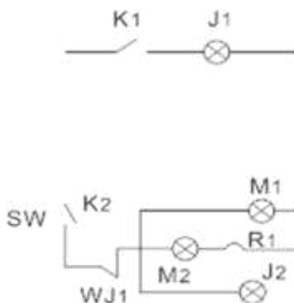
Рисунок 4: Схема электроподключения
