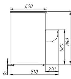
НЕЙТРАЛЬНЫЙ ПРИЛAVOK
