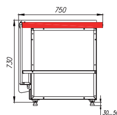
НЕЙТРАЛЬНЫЙ ПРИЛAVOK
