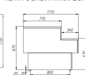
НЕЙТРАЛЬНЫЙ ПРИЛАВОК
