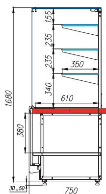
НЕЙТРАЛЬНАЯ БАШНЯ
