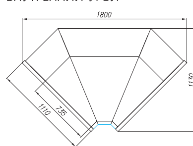
ВНУТРЕННИЙ УГОЛ
