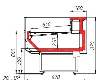
СТАТИЧЕСКАЯ ОТКРЫТАЯ
