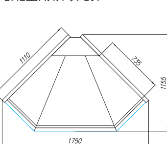
ВНЕШНИЙ УГОЛ
