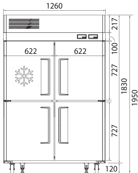
ВИД СПЕРЕДИ
