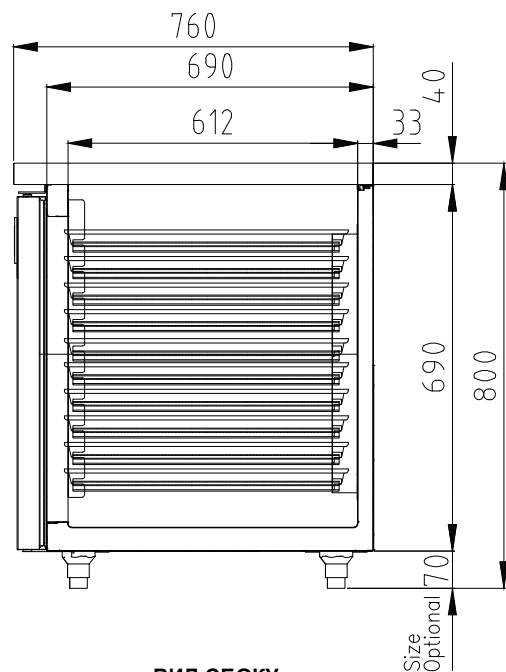
ВИД СБОКУ
