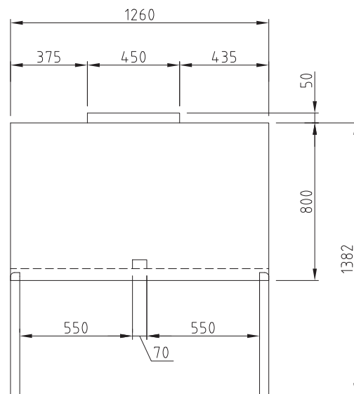
ВИД СВЕРХУ
