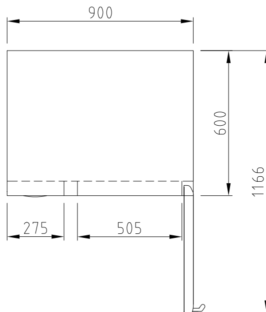
ВИД СВЕРХУ
