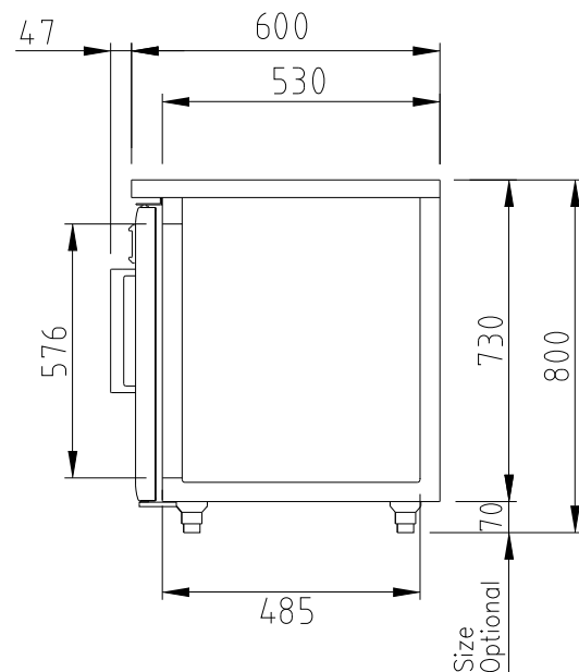
ВИД СБОКУ
