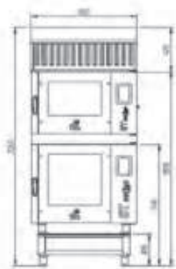
CAMPANA ST ST 604 ST 606 SOPORTE ST 300 KIT SUPERPOSICIÓN SERIE ST
