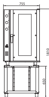
RXB 616 SOPORTE RXB 650
