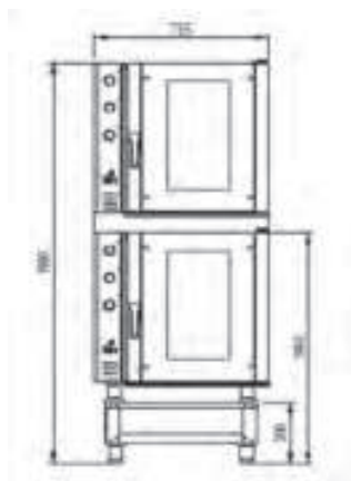
RXB 606 RXB 606 SOPORTE RXB300 300 KIT SUPERPOSICIÓN SERIE RXB
