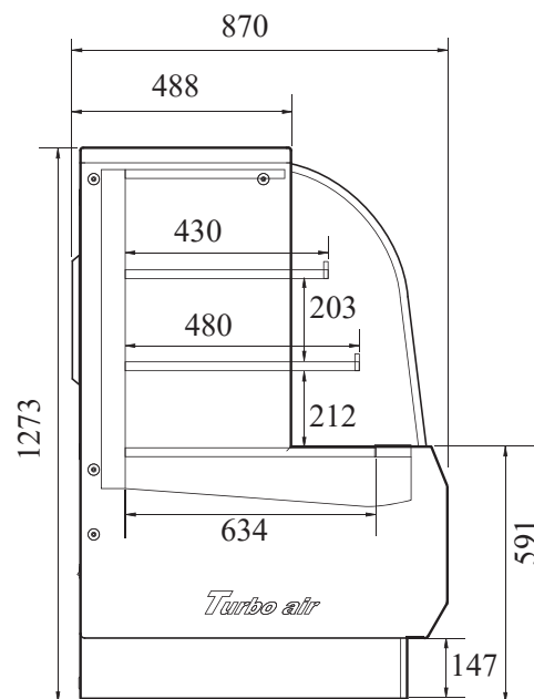
ВИД СБОКУ
