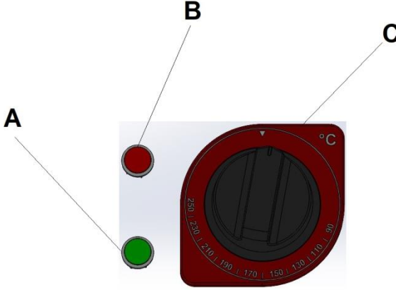
Şekil 1 Kontrol panosu
