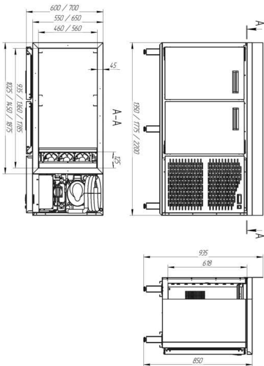
Стол холодильный КСХ (КСМ) с боковым расположением агрегата
