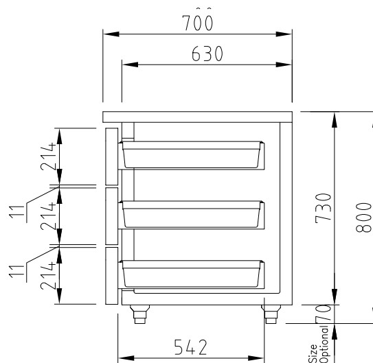
ВИД СБОКУ
