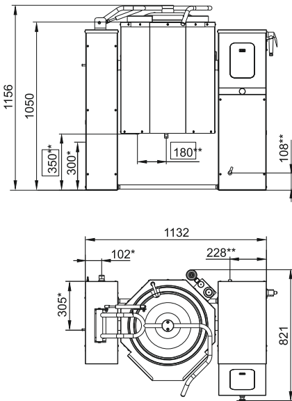
КПЭМ-60-О
