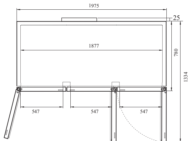
ВИД СВЕРХУ
