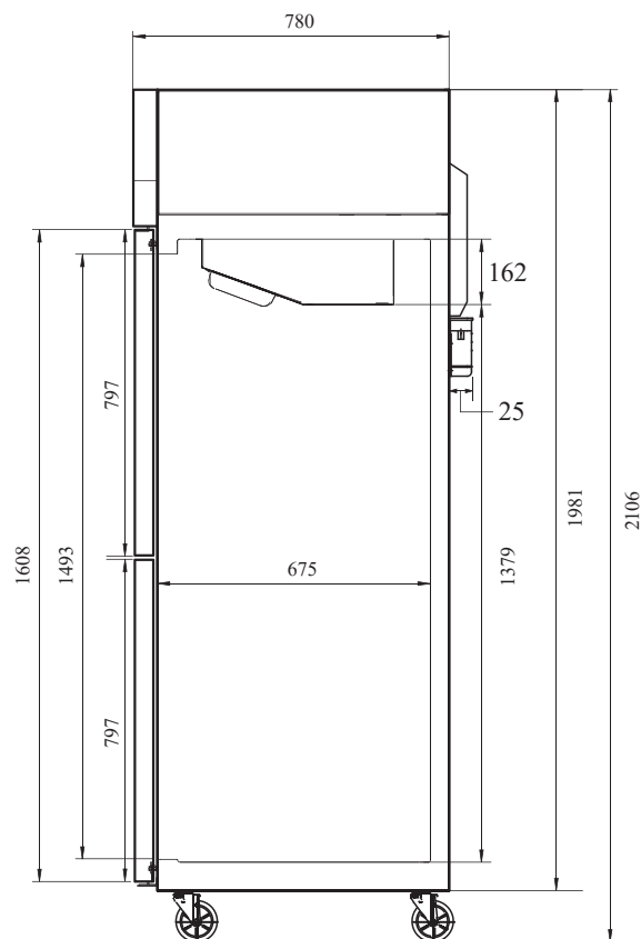
ВИД СБОКУ
