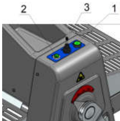
Рис. 4 - Панель управления
