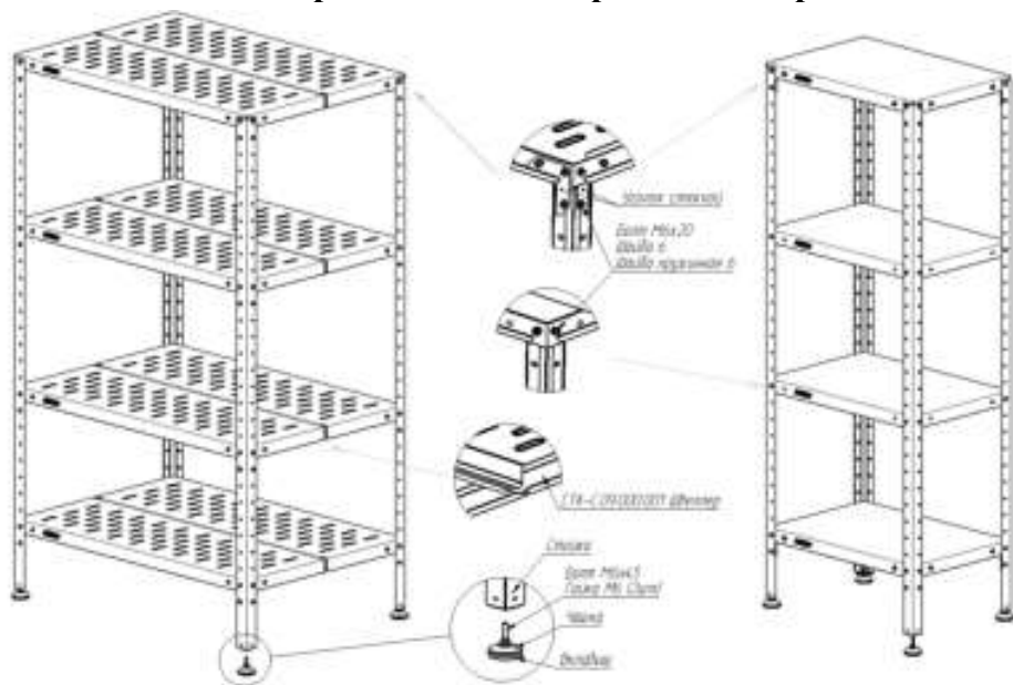
Схема сборки стеллажей серии «Стандарт»
