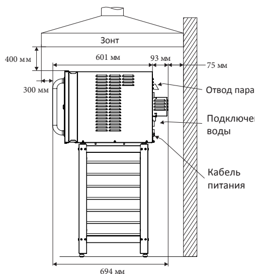
ВИД СБОКУ
