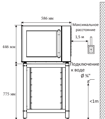
ВИД СПЕРЕДИ
