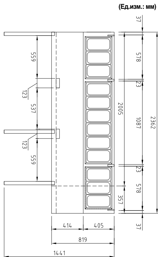
ВИД СВЕРХУ
