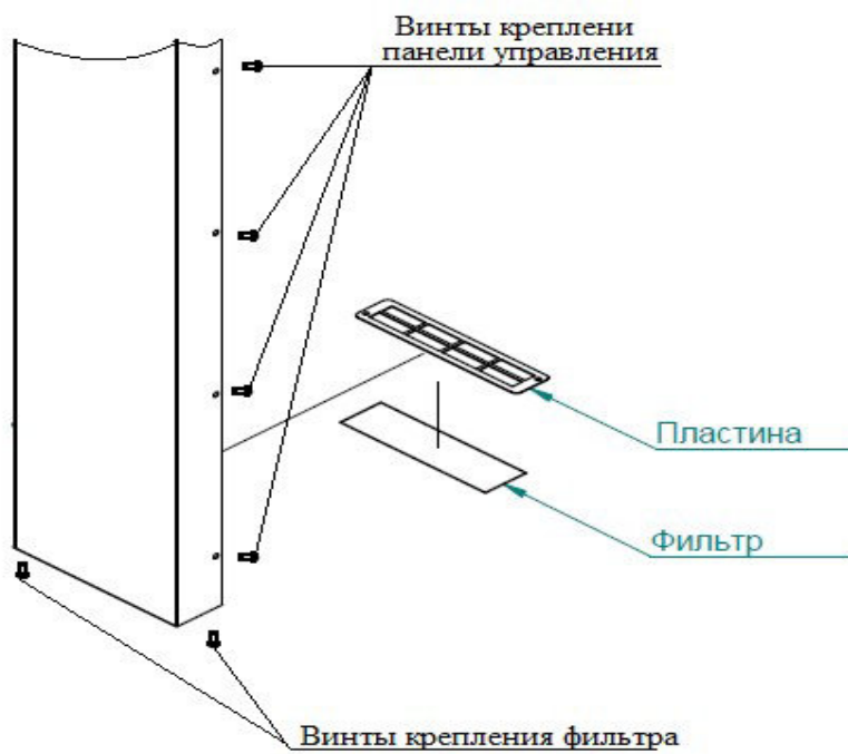
Рис. 17. Замена фильтра
