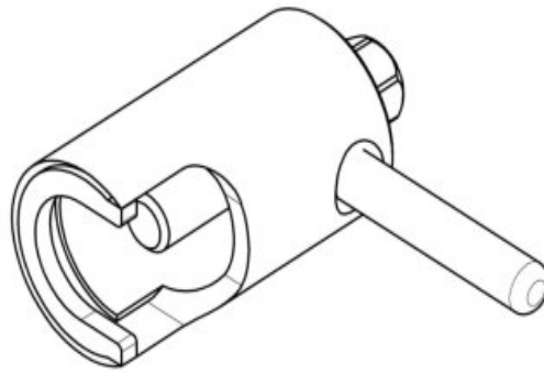
Рис. 11. Съемник крыльчатки.
