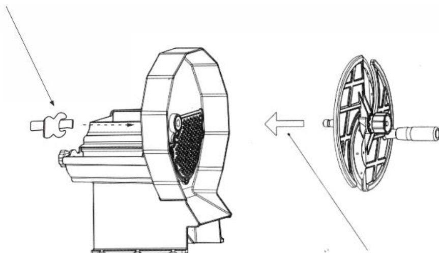
Рис 2. Сборка слайсера
