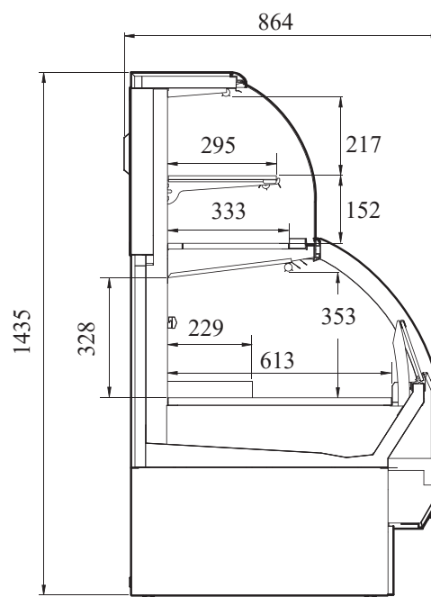
ВИД СБОКУ
