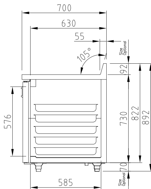
ВИД СБОКУ
