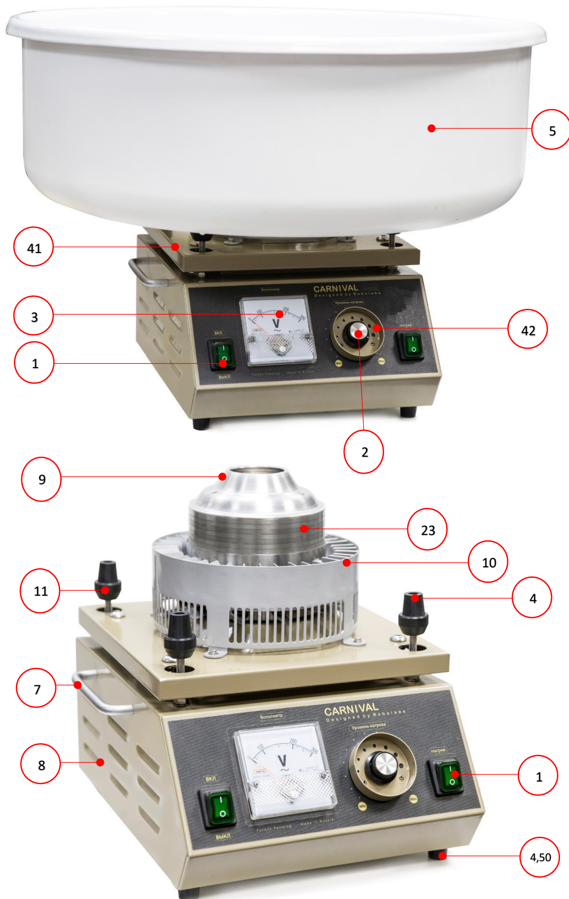
Общий вид для ТМ 2620-00, ТМ 2620-04, ТМ 3677-00 и ТМ 3677-04
