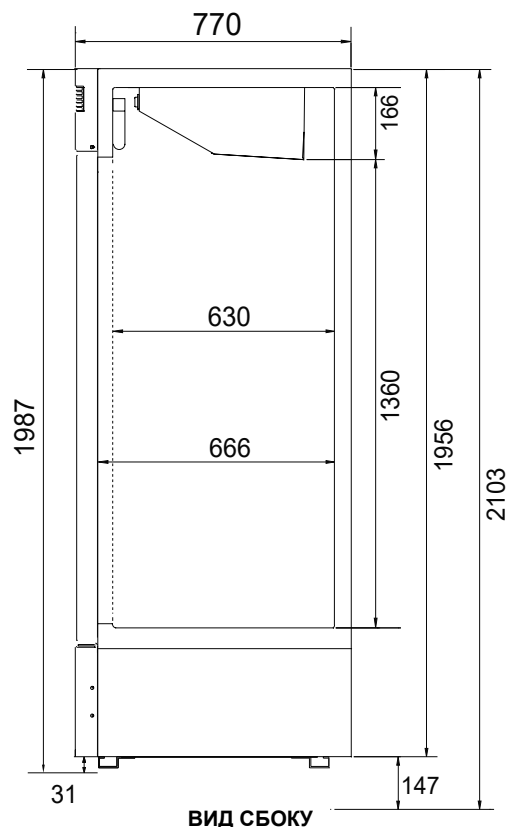
ВИД СБОКУ
