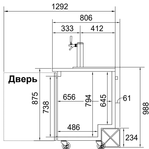
ВИД СБОКУ
