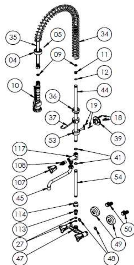
Installation Diagram for MT04 Схема установки для MT04
