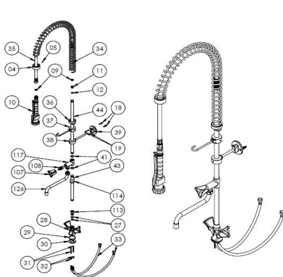
Installation Diagram for MT02 Схема установки для MT02
