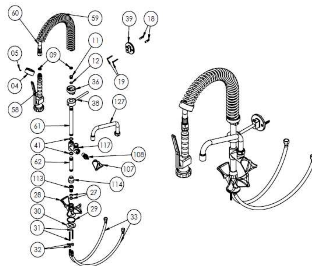
Installation Diagram for MT06 Схема установки для MT06
