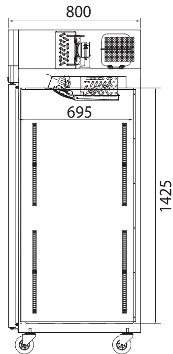
ВИД СБОКУ
