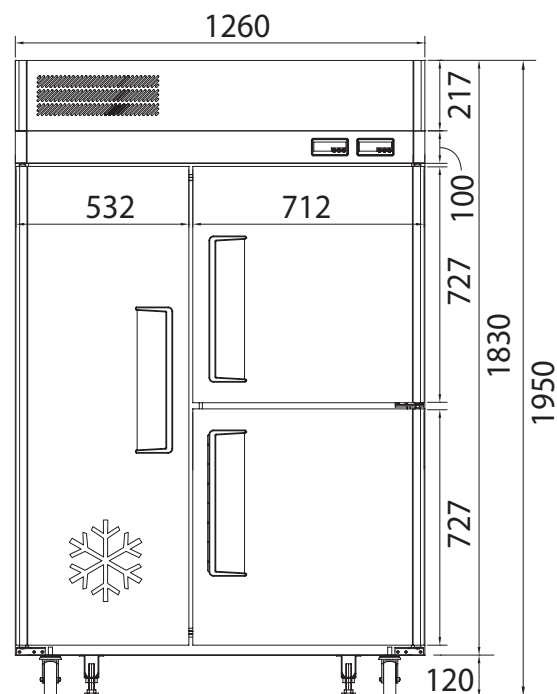
ВИД СПЕРЕДИ
