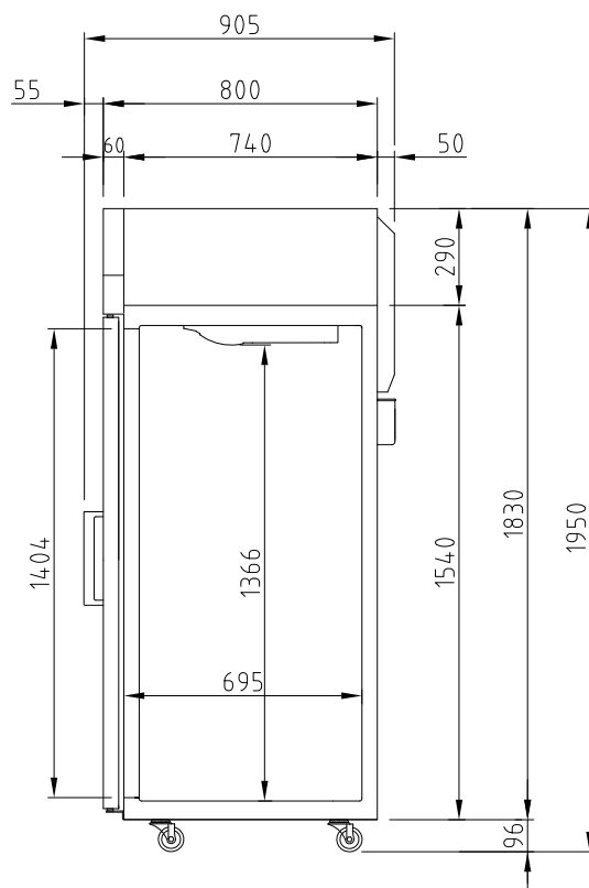
ВИД СБОКУ
