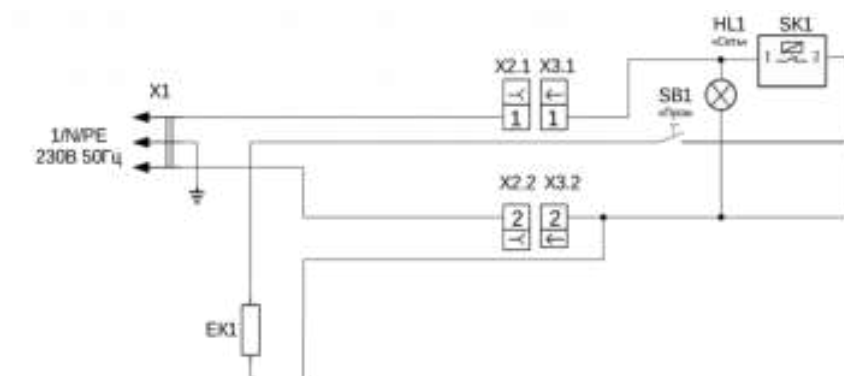
Схема электрическая принципиальная ШРТ 8
