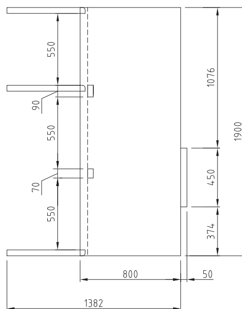
ВИД СВЕРХУ
