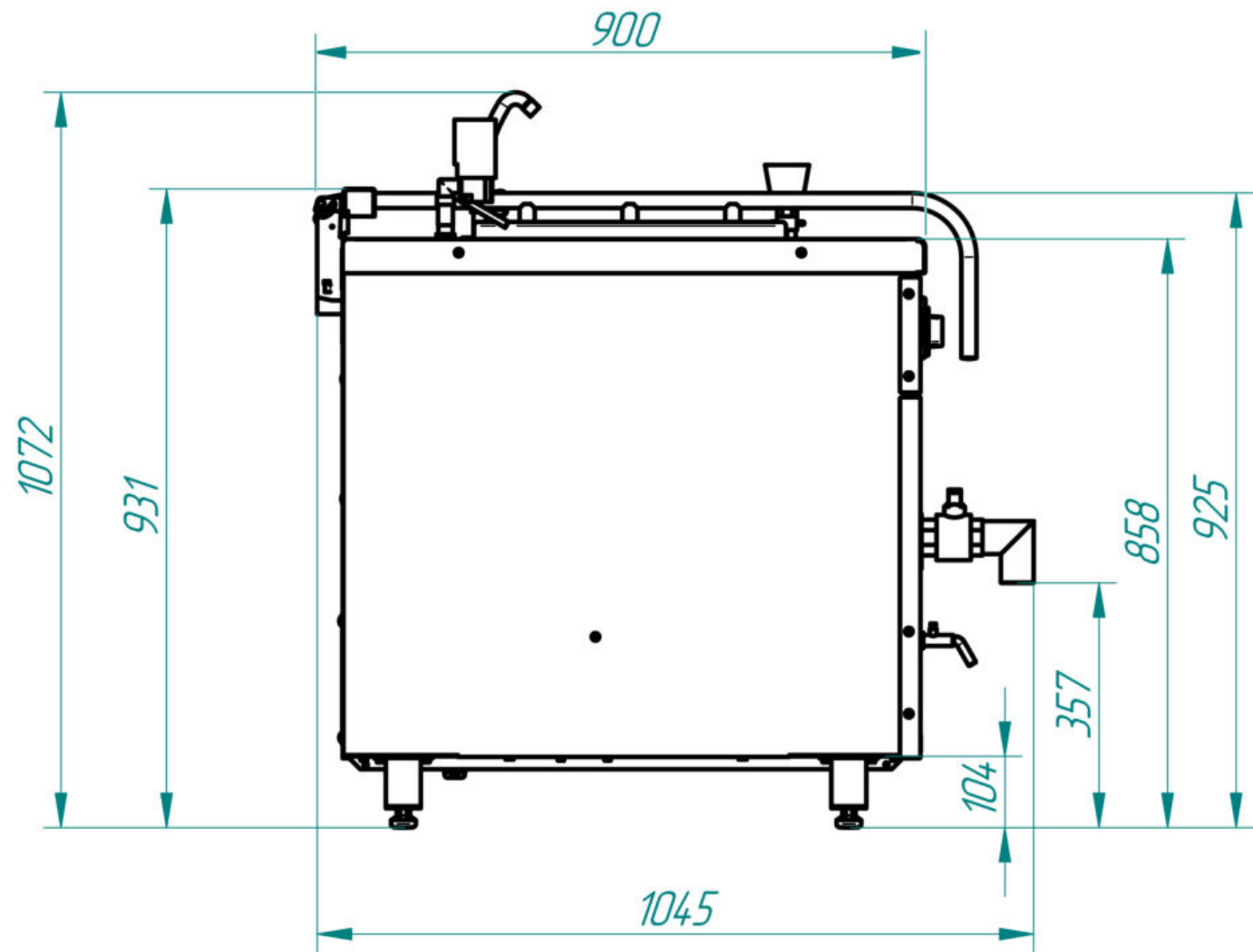
КПЭ-60.00.00.000 СБ _ Котел пищеварочный КПЭ-60-М
