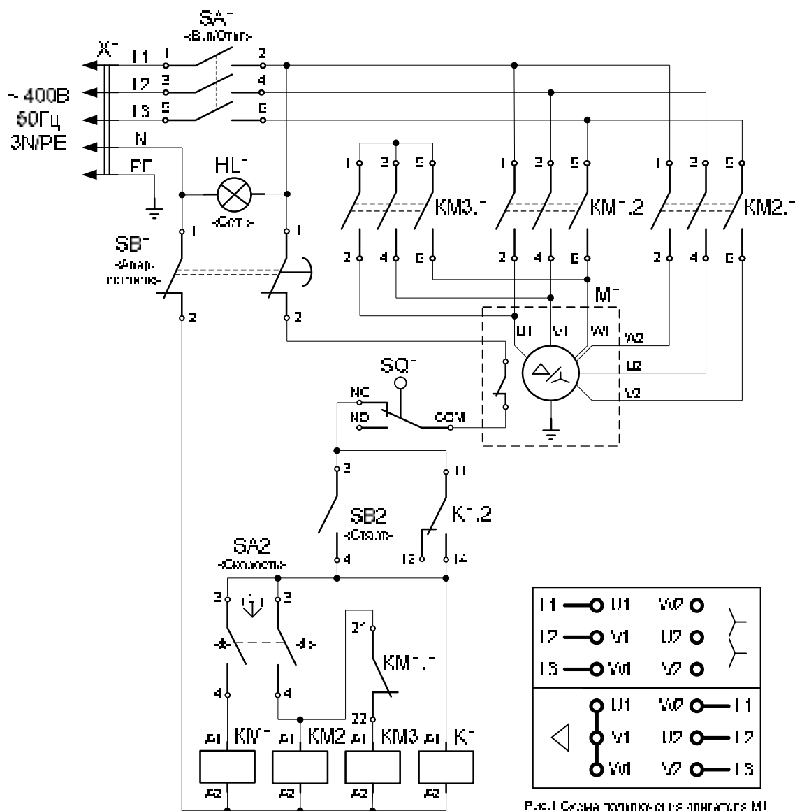
Рис.1 Схема подключения двигателя M1
