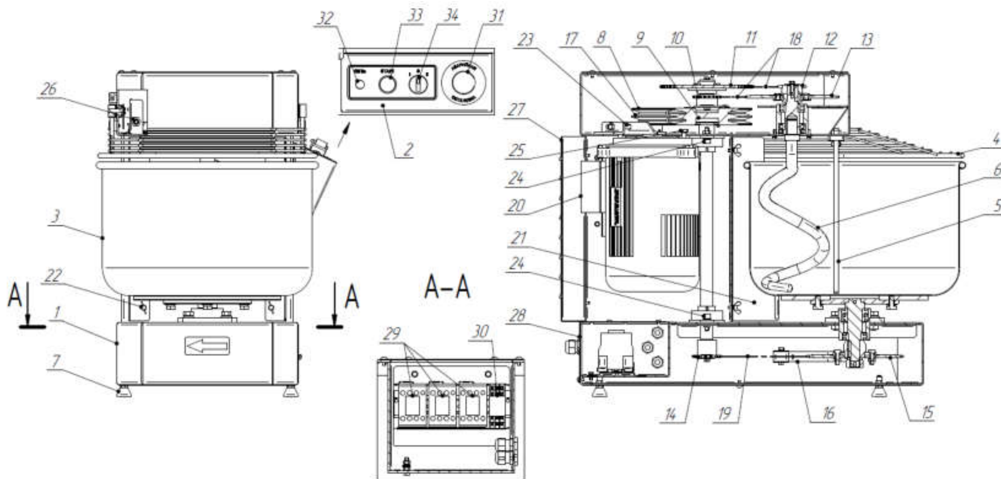
1. Корпус; 2. Панель управления; 3. Дежа; 4. Защитная решетка дежи; 5. Нож; 6. Месильный орган (спираль); 7. Ножка; 8. Шкив малый; 9. Шкив большой; 10. Звездочка малая; 11. Звездочка большая; 12. Звездочка малая; 13. Звездочка большая; 14. Звездочка малая (нижняя); 15. Звездочка большая (нижняя); 16. Натяжитель; 17. Ремень; 18. Цепи верхние; 19. Цепь нижняя; 20. Электродвигатель; 21. Защитный кожух; 22. Винт-барашек; 23. Болт натяжения ремня(-ей); 24. Винты фиксации промежуточного вала; 25. Болты фиксации электродвигателя; 26. Микровыключатель; 27. Задняя стенка; 28. Крышка; 29. Контактор; 30. Реле; 31. Кнопка «Аварийная остановка»; 32. Лампа «Сеть»; 33. Кнопка «Старт»; 34. Переключатель «Скорость».
