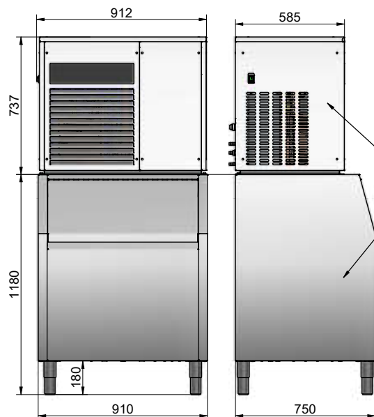
Льдогенератор ЛГ-620Ч-01/-02
