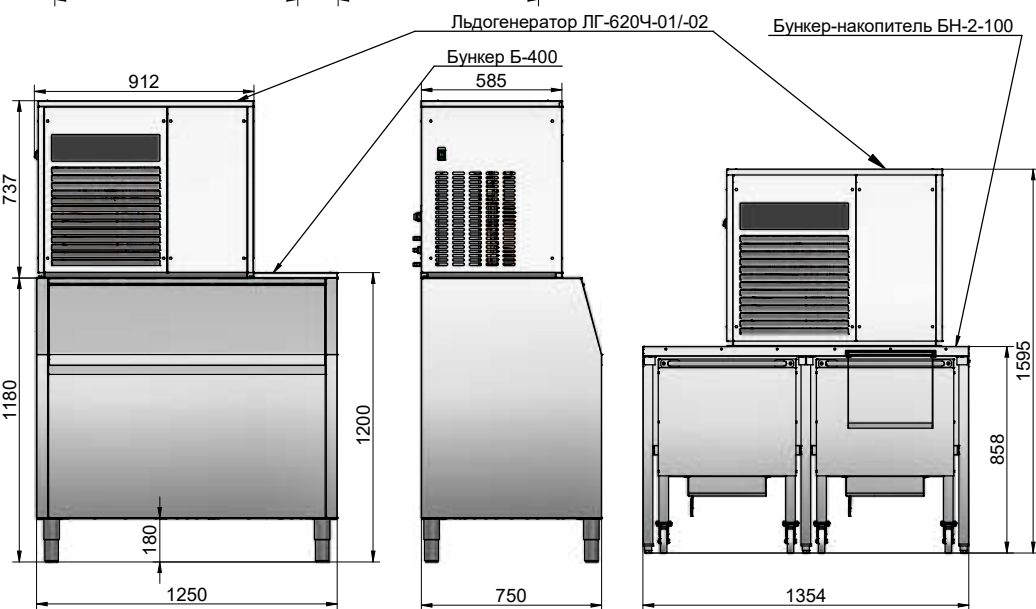
Льдогенератор ЛГ-620Ч-01/-02
