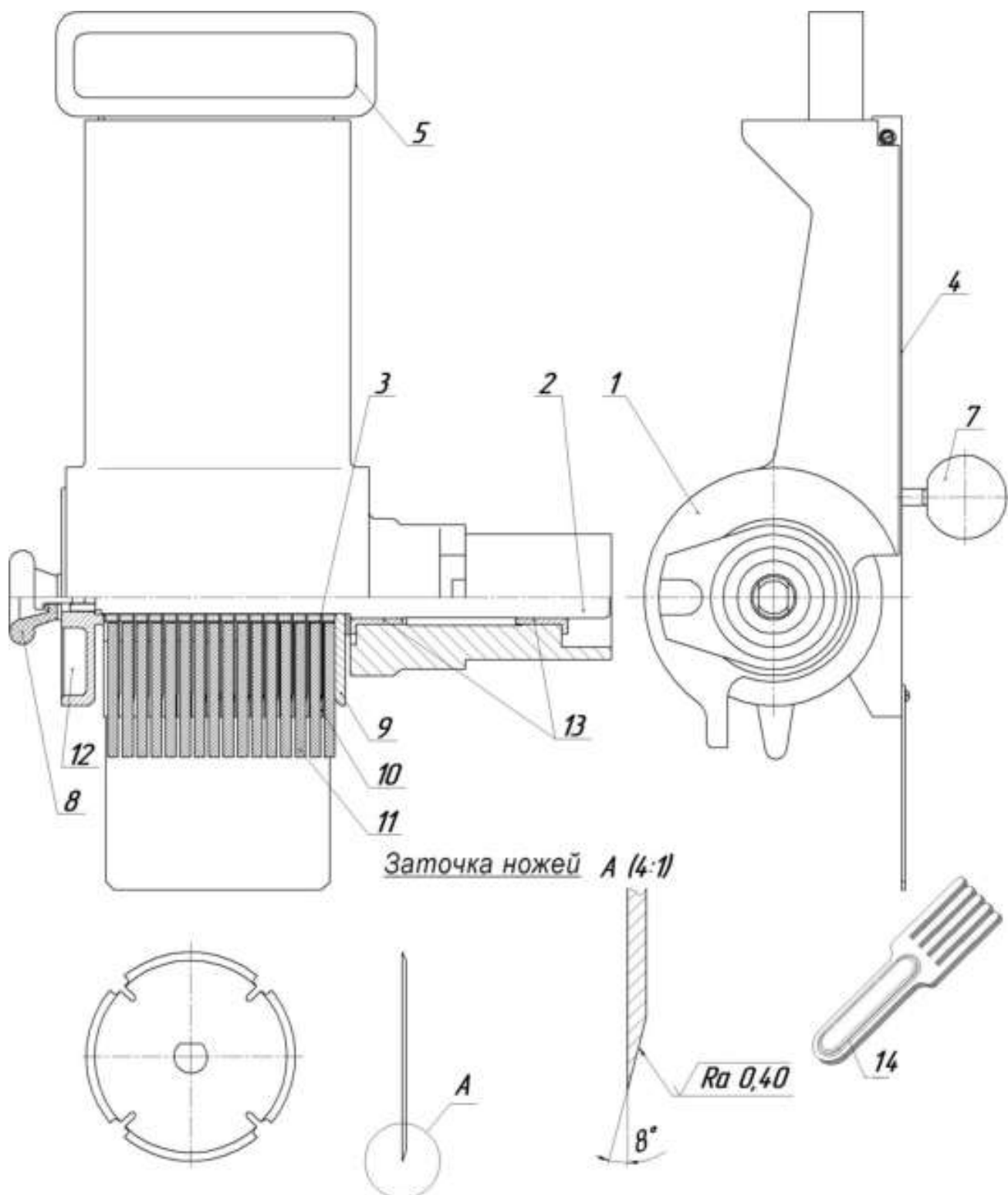
Рисунок 25 – Механизм для нарезания мяса на бефстроганов 1 - корпус, 2 - вал ножевой, 3 – кольцо, 4 – заслонка, 5 - толкатель, 7 - ручка, 8 - рукоятка, 9 – диск, 10 – фреза, 11 - упор, 12 - диск, 13 – втулка, 14 – прочистка.
