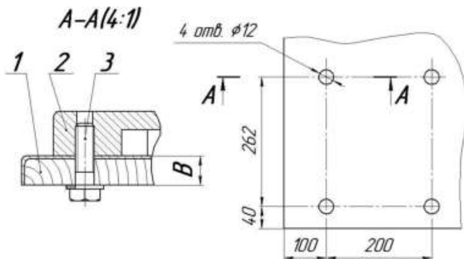
Рисунок 27 – Схема установки приводного механизма на столе
