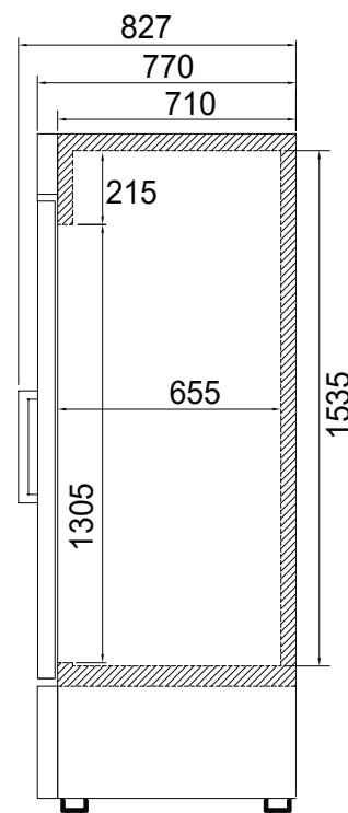
ВИД СБОКУ
