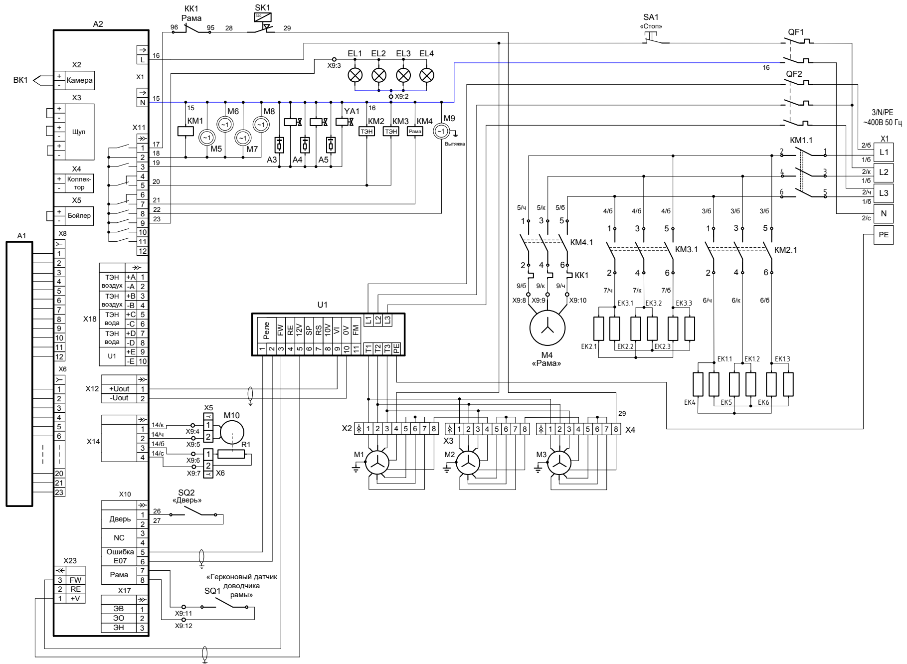
Рис.6 СХЕМА ЭЛЕКТРИЧЕСКАЯ ПРИНЦИПИАЛЬНАЯ РПШ-18-8-6МР
